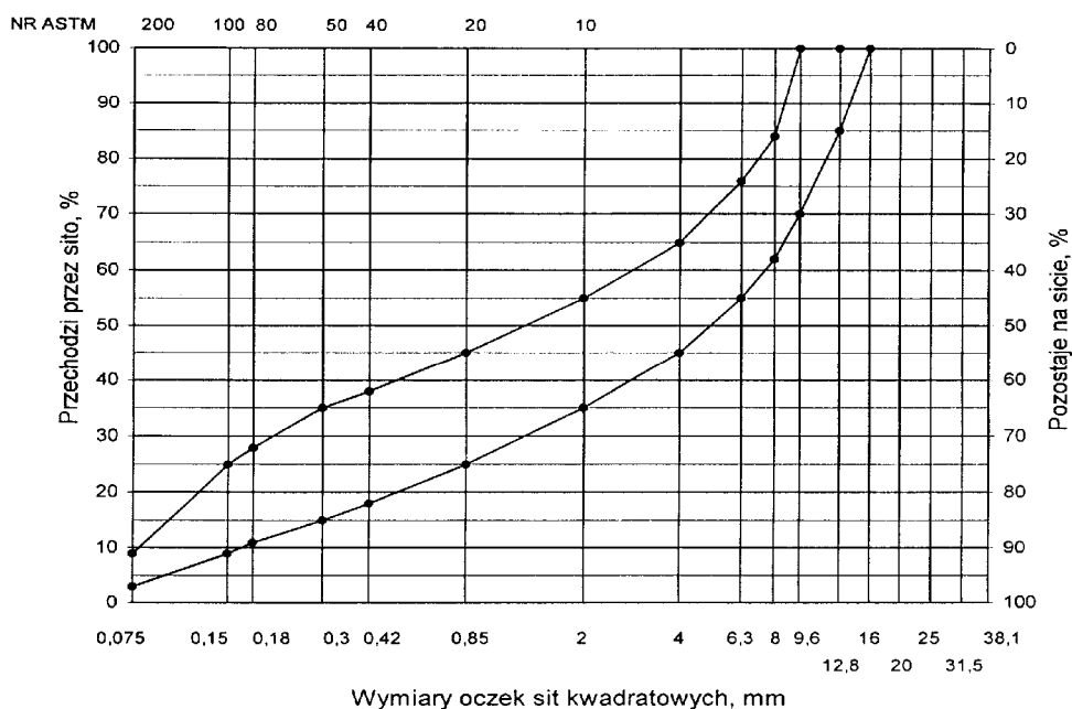
Rys. 3. Krzywe graniczne uziarnienia mieszanki mineralnej BA od 0 do 12,8 mm do warstwy wiążącej i wyrównawczej, nawierzchni drogi o obciążeniu ruchem KR1 lub KR2
